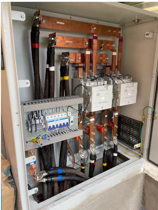
Foto 3: Quadro de Transferência Automática do gerador perto do poste.
